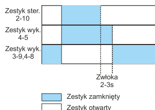
Diagram pracy
